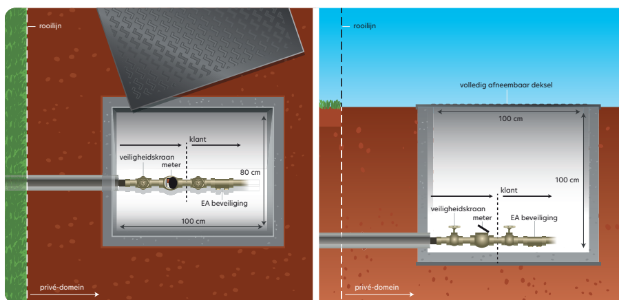
Dit schema toont het bovenaanzicht van een aftakking met diameter 32.
