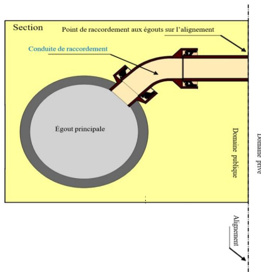
Figure 1 - Schéma de principe du raccordement à un conduit d'égout
